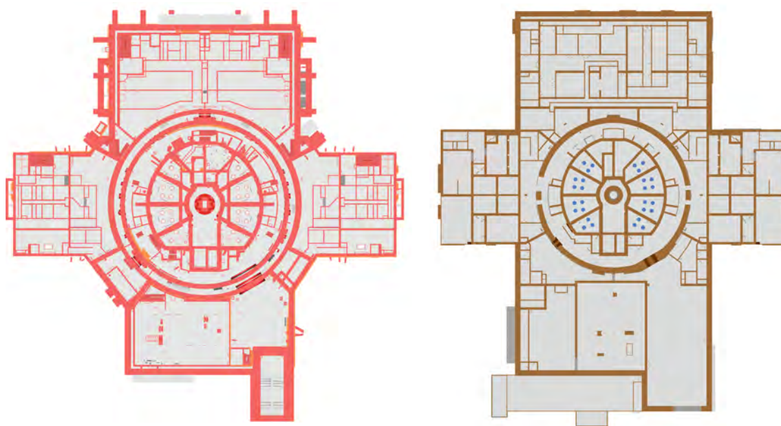
Comparaison de la structure des bâtiments entre un EPR (à gauche) et un EPR2 (à droite).
